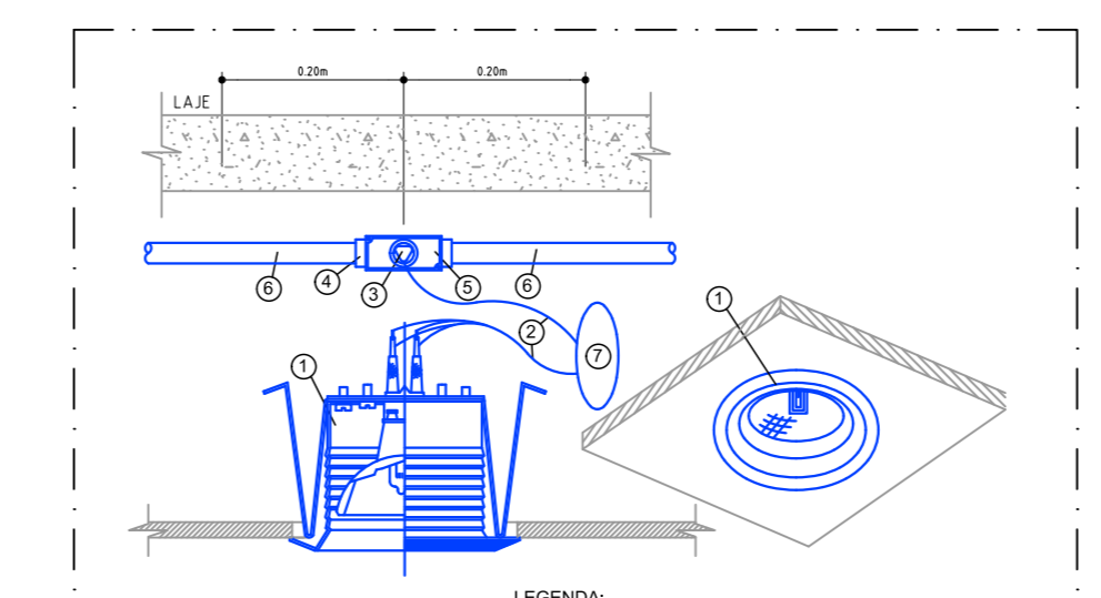
DETALHE - 002 LUMINÁRIA EMBUTIDA EM FORRO SEM ESCALA
