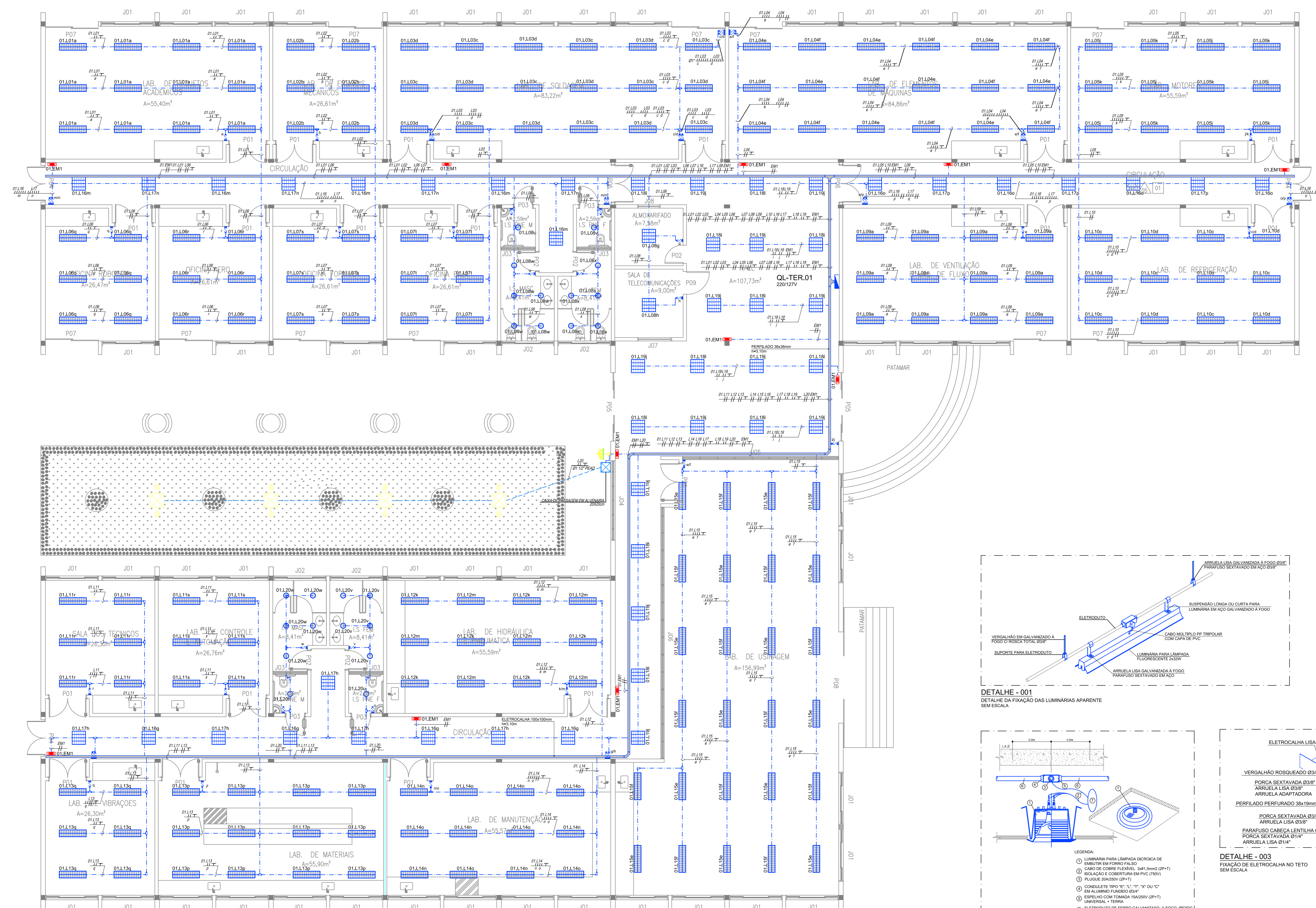
PLANTA - TÉRREO ESC. 1/75
