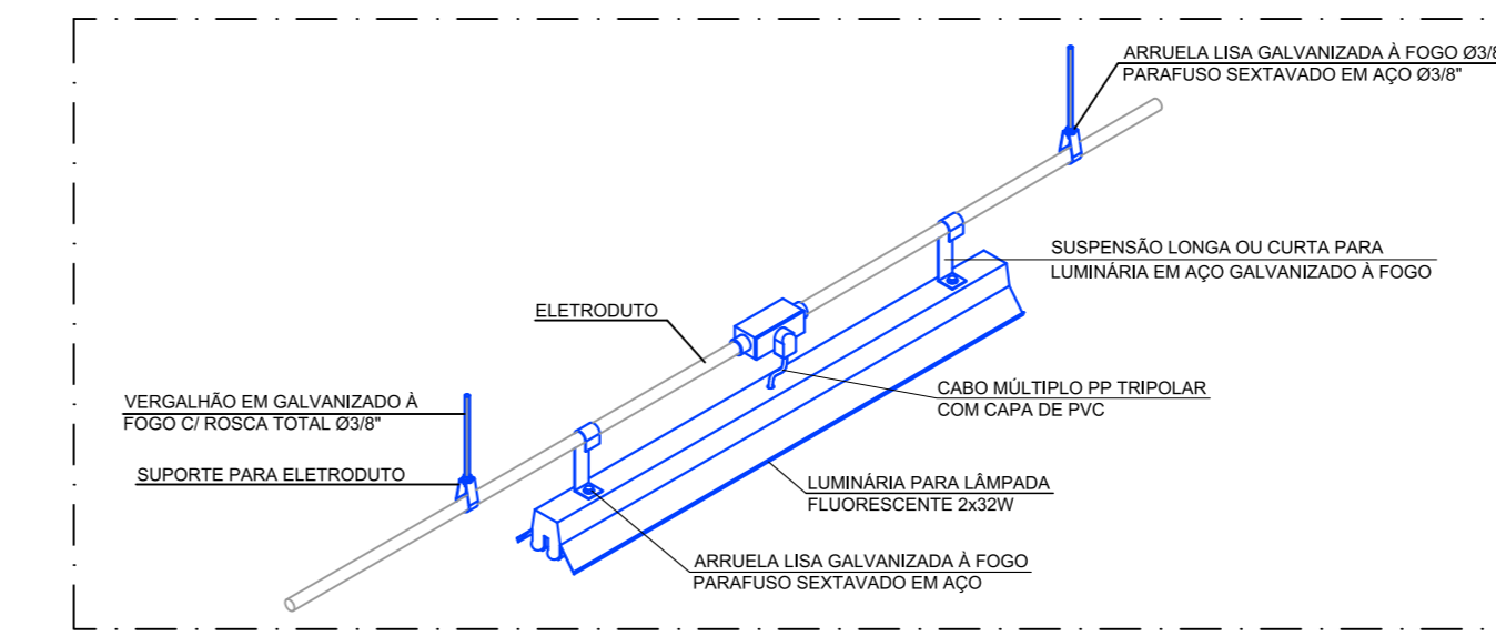
DETALHE - 001 DETALHE DA FIXAÇÃO DAS LUMINÁRIAS APARENTE SEM ESCALA
