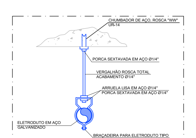
DETALHE - 002 FIXAÇÃO DE ELETRODUTO SEM ESCALA
