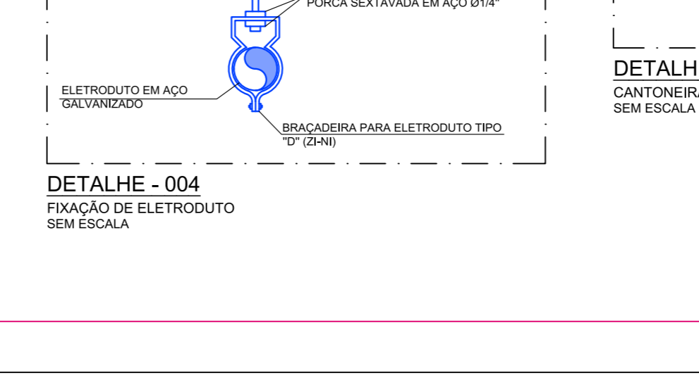
DETALHE - 004 FIXAÇÃO DE ELETRODUTO SEM ESCALA
