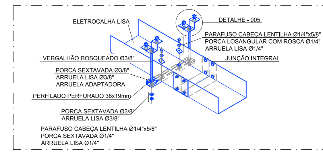
DETALHE - 005 ELETROCALHA LISA
