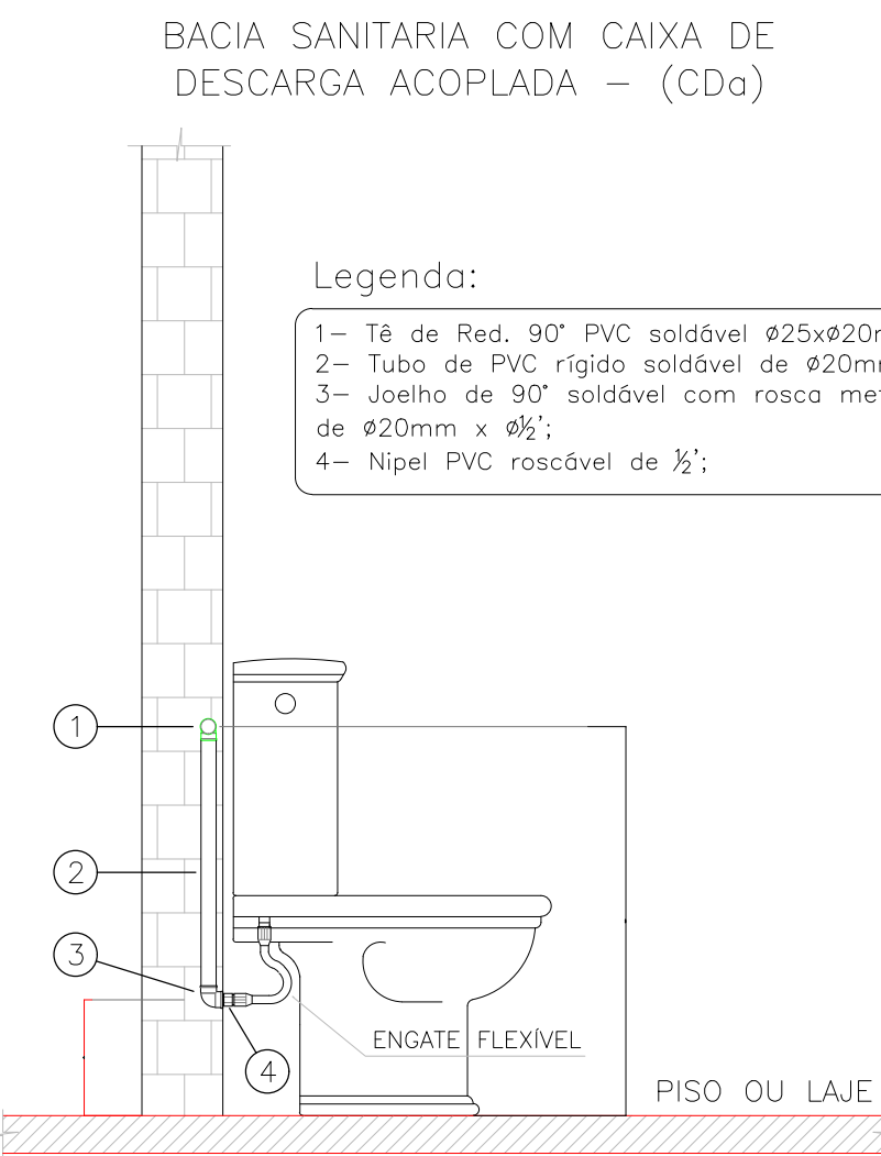
DET. DE MONTAGEM – LOUÇAS SANITÁRIAS SEM ESCALA
