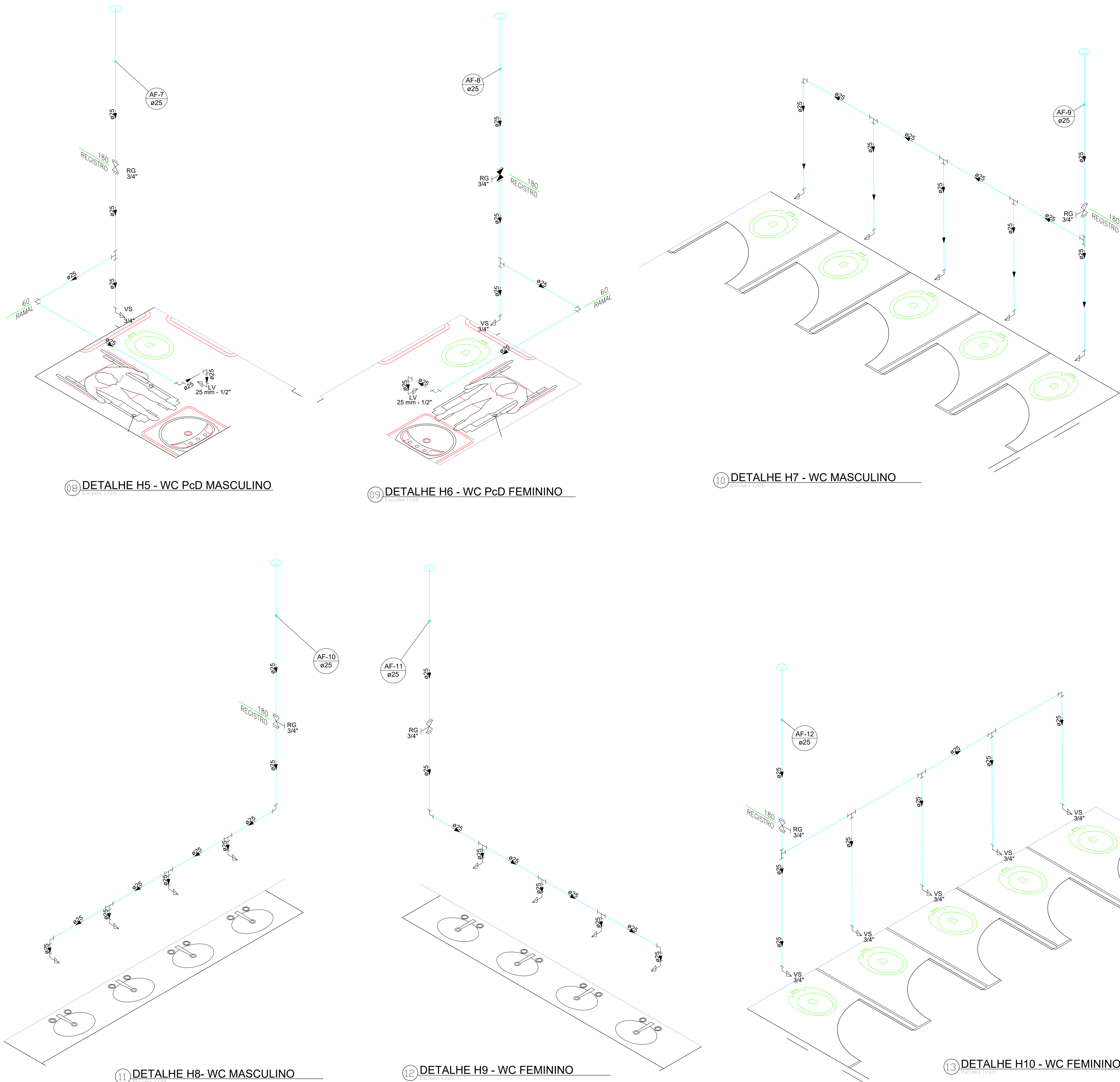
11.DETALHE H8 - WC MASCULINO
