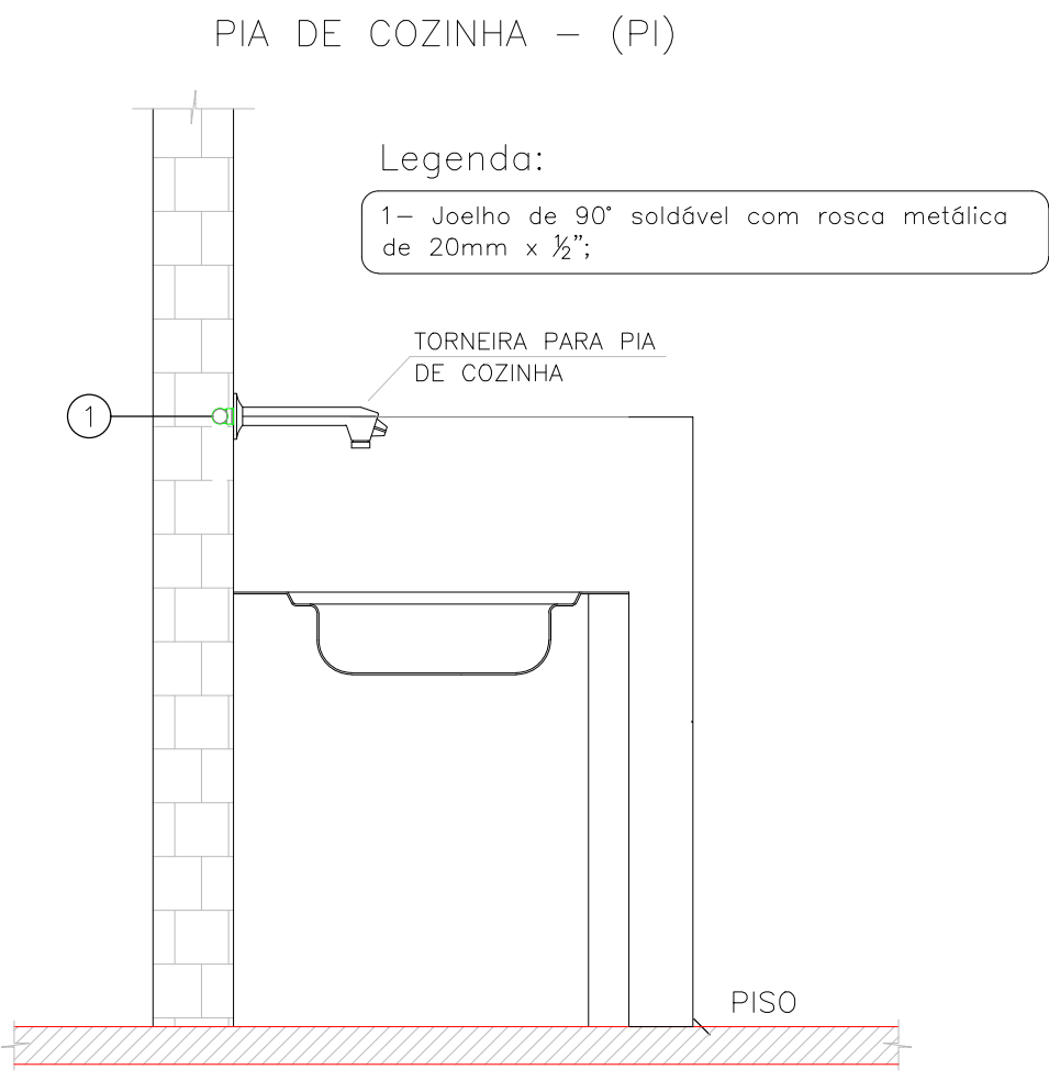
DET. DE MONTAGEM – ÁREA EXTERNA, COZINHA E SERVIÇO SEM ESCALA
