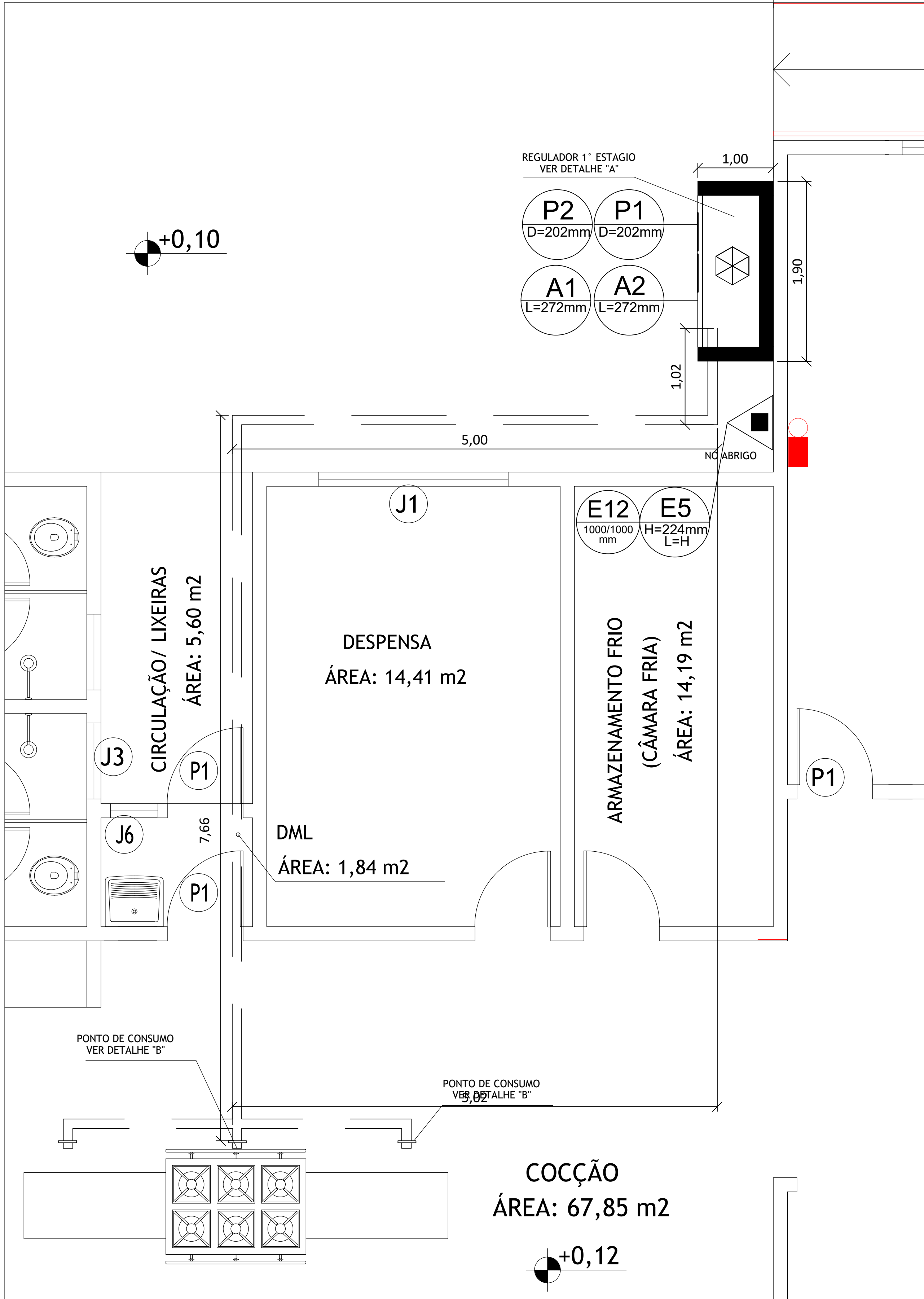
CENTRAL DE GLP - PLANTA BAIXA SEM ESCALA
