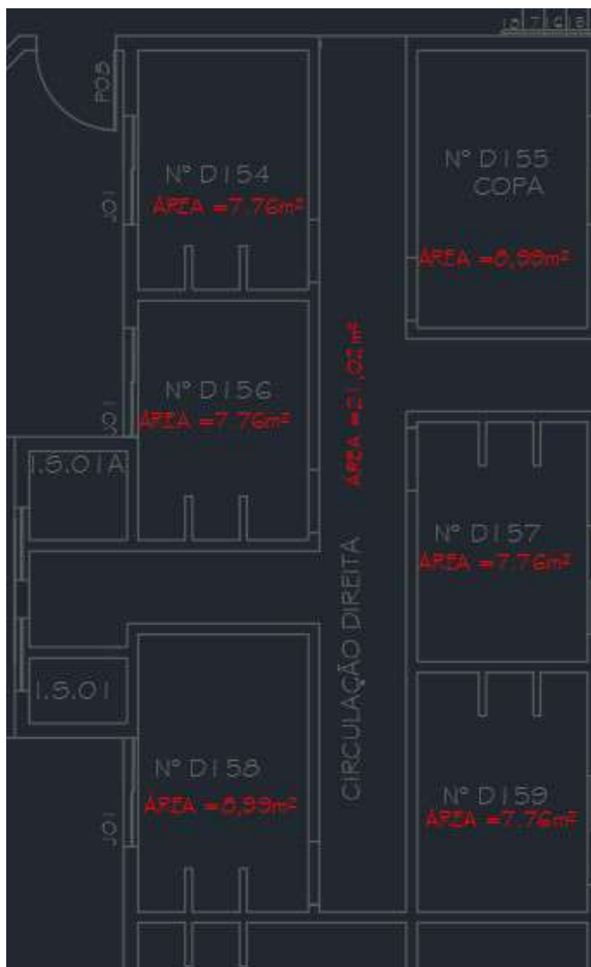
Foto 266: PLANTA BAIXA
