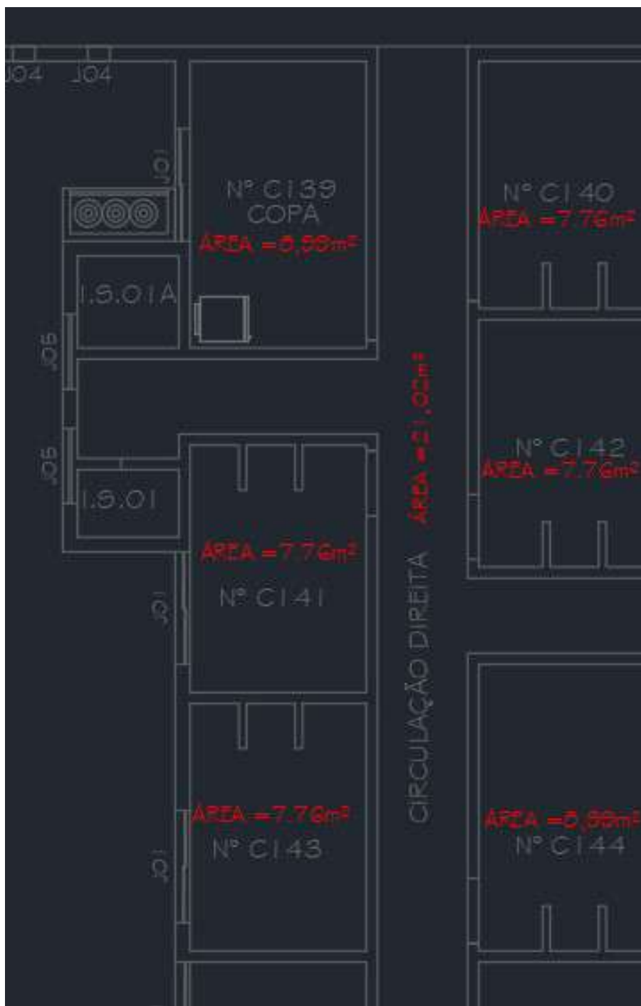
Foto 282: PLANTA BAIXA
