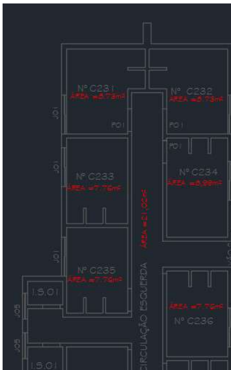
Foto 184: PLANTA BAIXA
