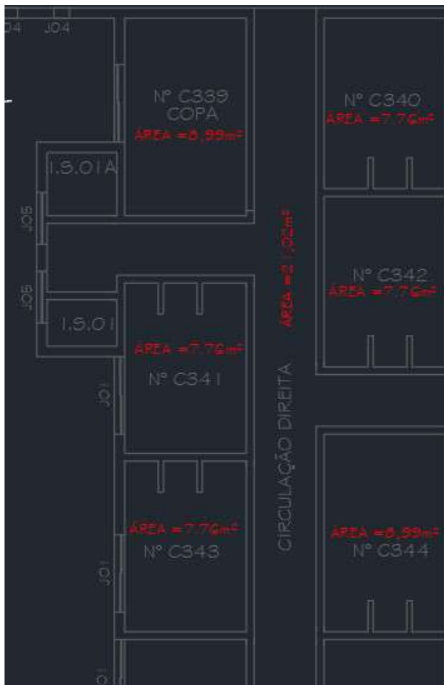
Foto 75: PLANTA BAIXA
