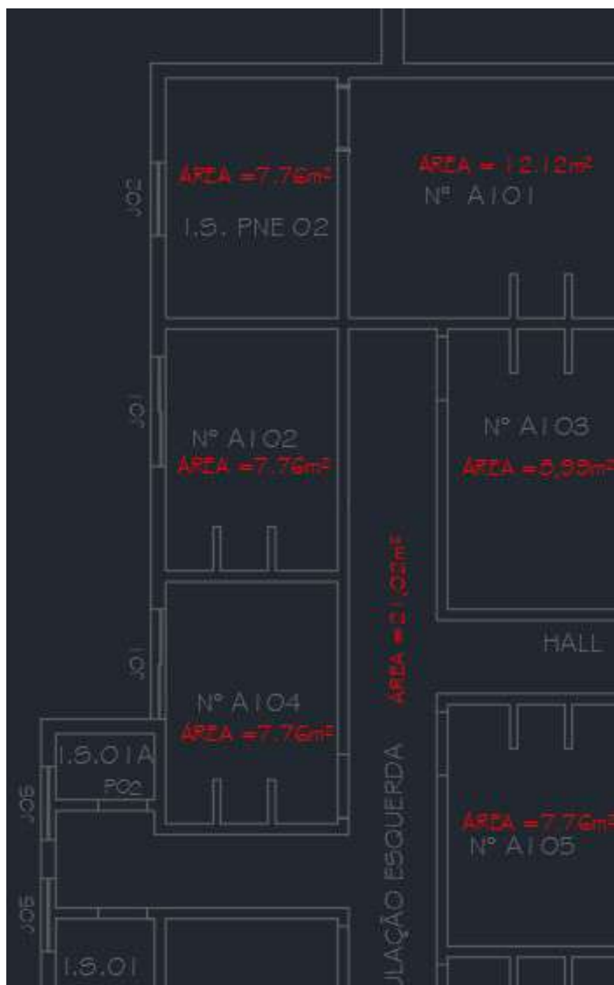
Foto 362: PLANTA BAIXA
