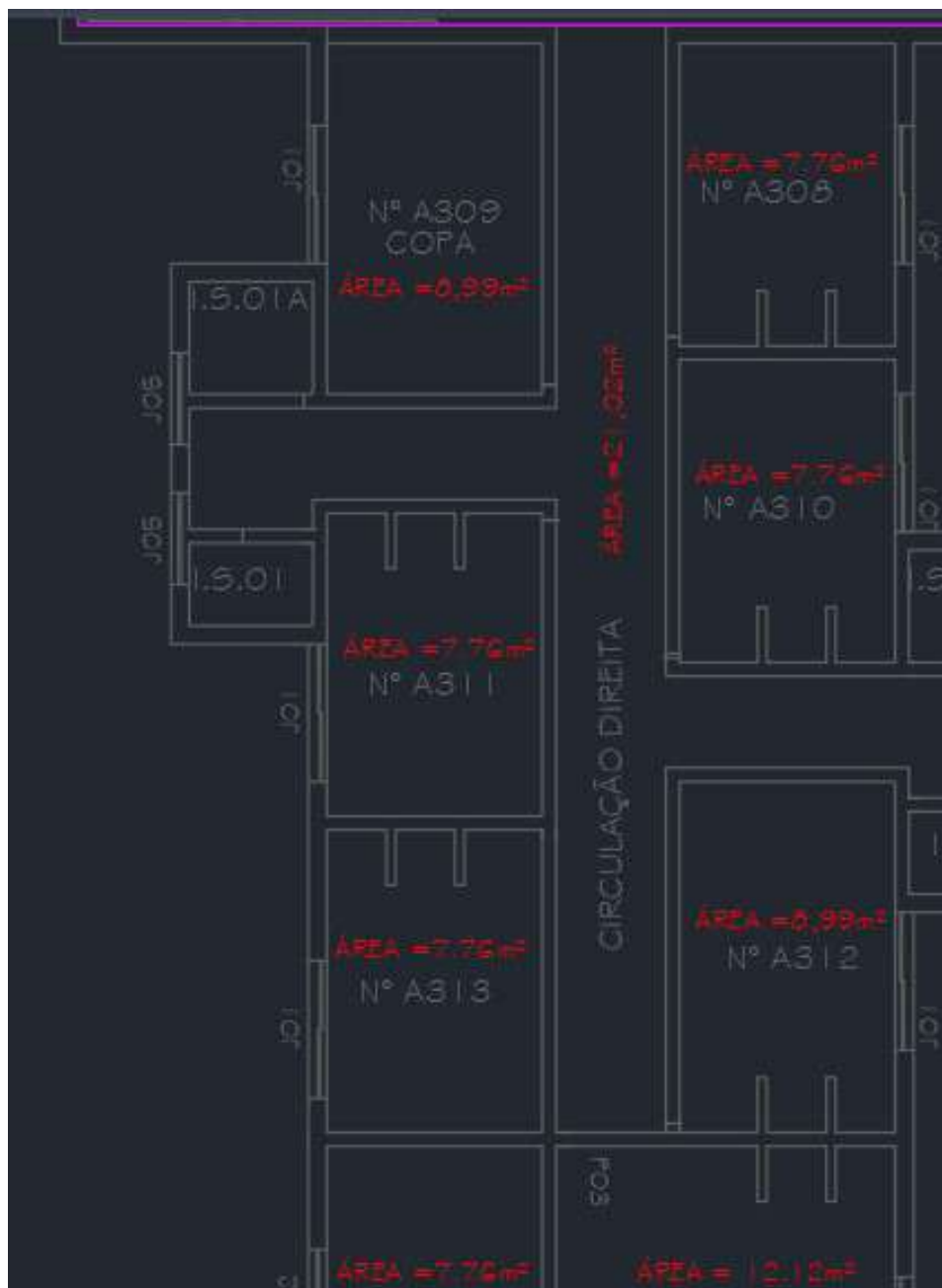
Foto 01: PLANTA BAIXA
